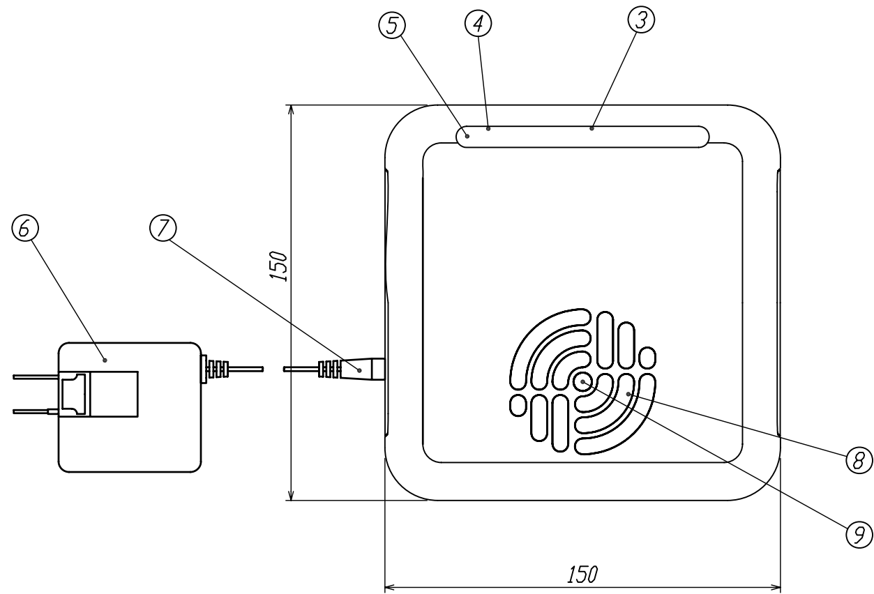
正面図
